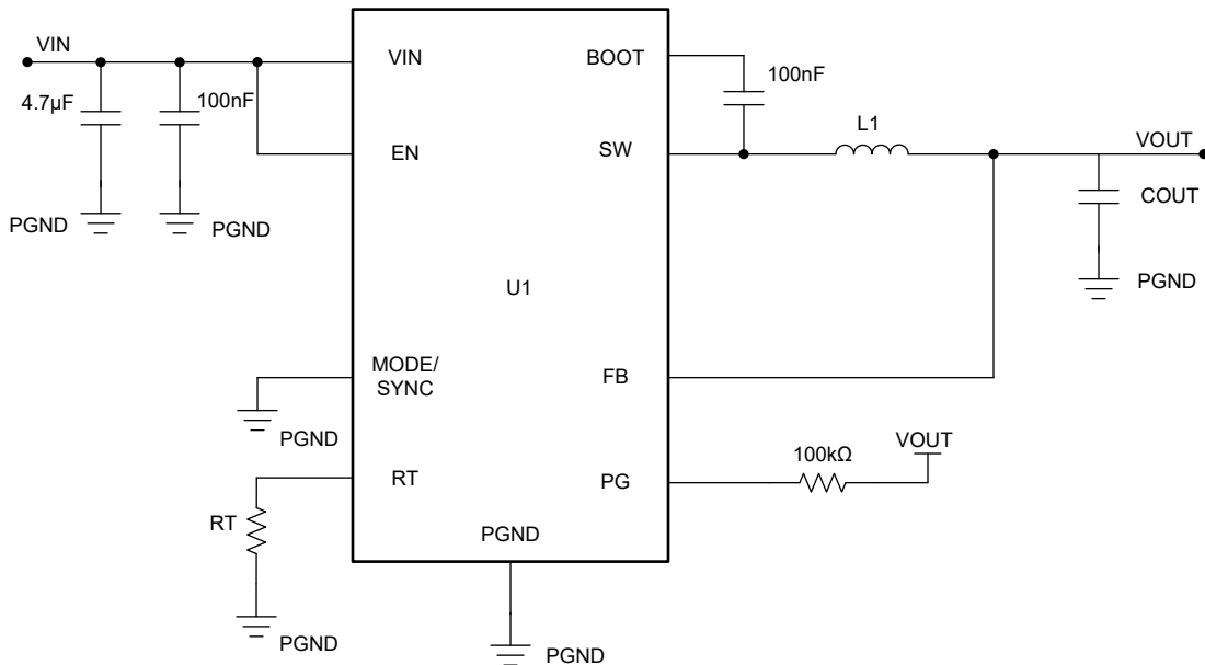
図 8-32. アプリケーション回路例
