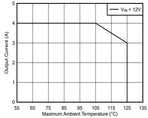
図 8-15. 出力電流と最大周囲温度との関係
