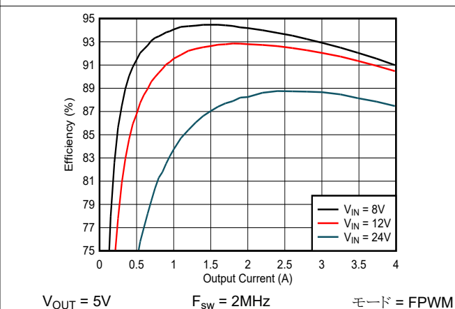
図 8-7. 効率
