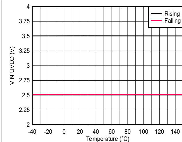
図 6-9. 入力電圧 UVLO 保護
