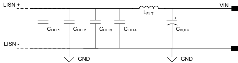
図 8-31. 標準入力 EMI フィルタ回路図
