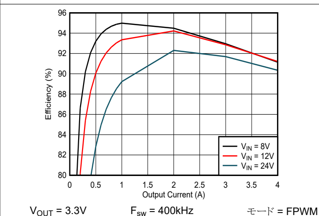
図 8-5. 効率
