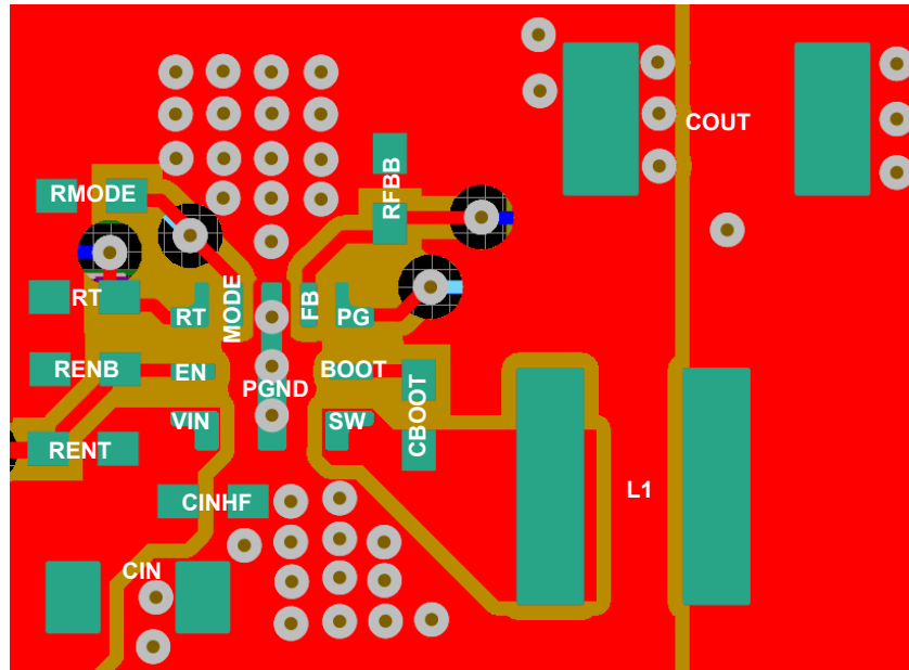
図 8-34. 固定出力バージョン
