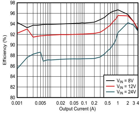
図 8-8. 効率
