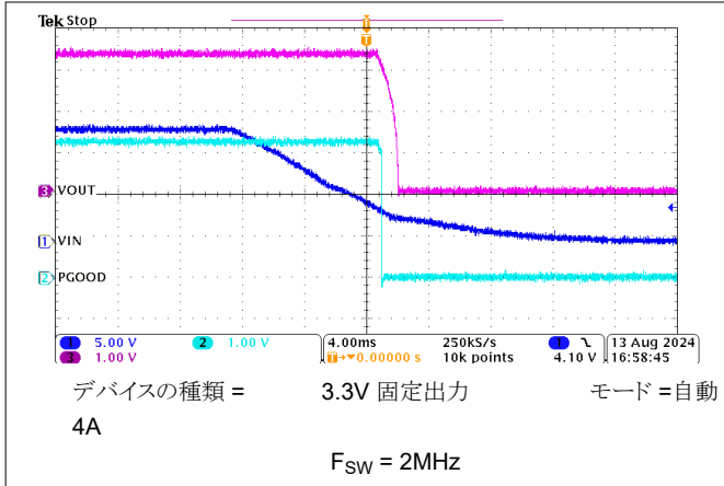
図 8-20. シャットダウン動作
