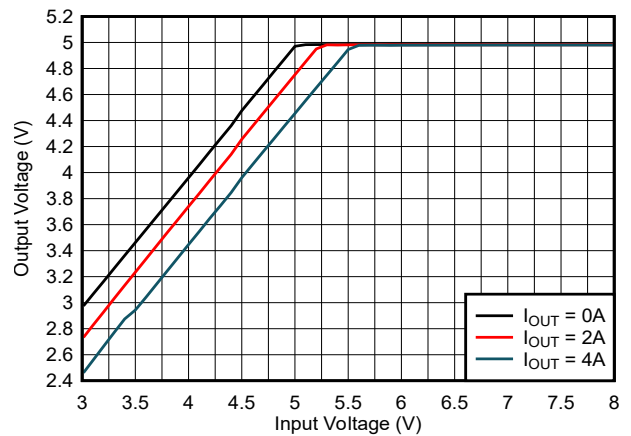
図 8-11. ドロップアウト
