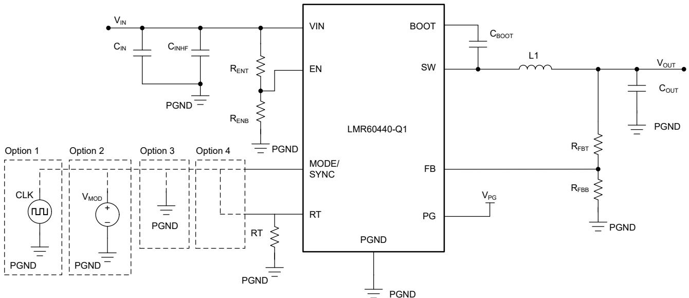
図 8-1. LMR60440-Q1 のリファレンス回路図
