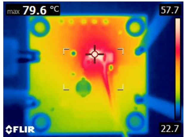
図 8-21. 短絡発生
