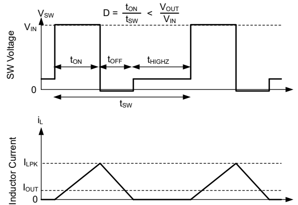
図 7-8. PFM 動作
