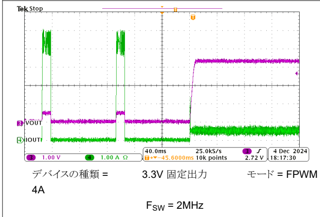
図 8-22. 短絡からの回復
