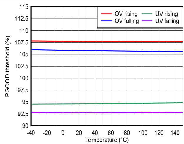
図 6-10. PGOOD スレッシュホールド
