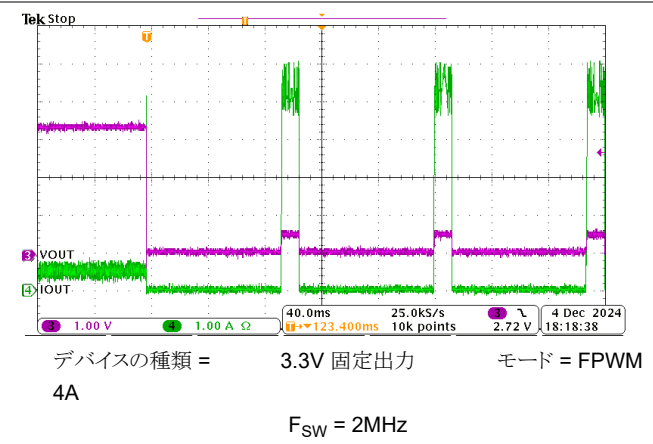
図 8-21. 短絡発生
