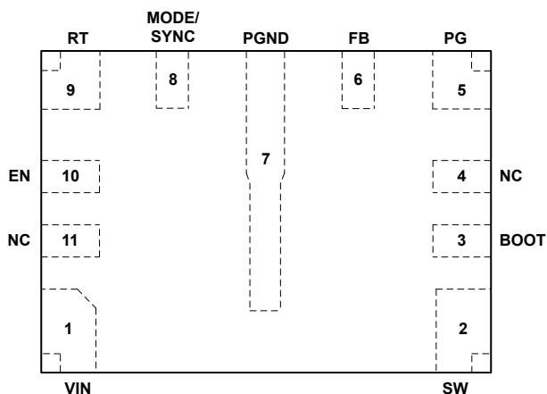
図 5-2. RBM パッケージ 11 ピン WQFN-HR (上面図)
