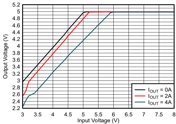
図 8-12. ドロップアウト
