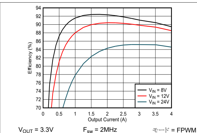
図 8-3. 効率
