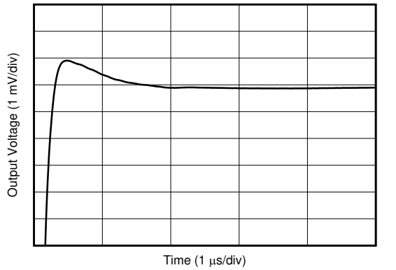
図 5-27. 大信号セトリング・タイム (正)
