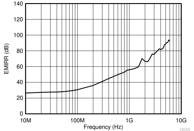
図 5-30. 非反転入力を基準とする電磁干渉除去比 (EMIRR+) と周波数との関係
