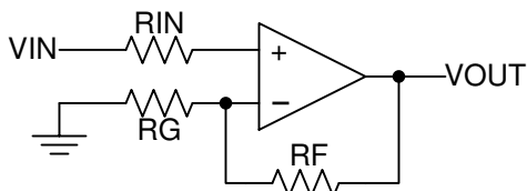
図 9-2. 非反転構成のオペアンプの回路図
