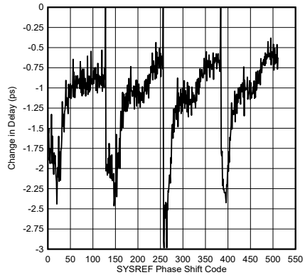
图 5-16. SYSREF Delta Delay vs. Code
