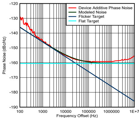
5-6. Flicker Noise
