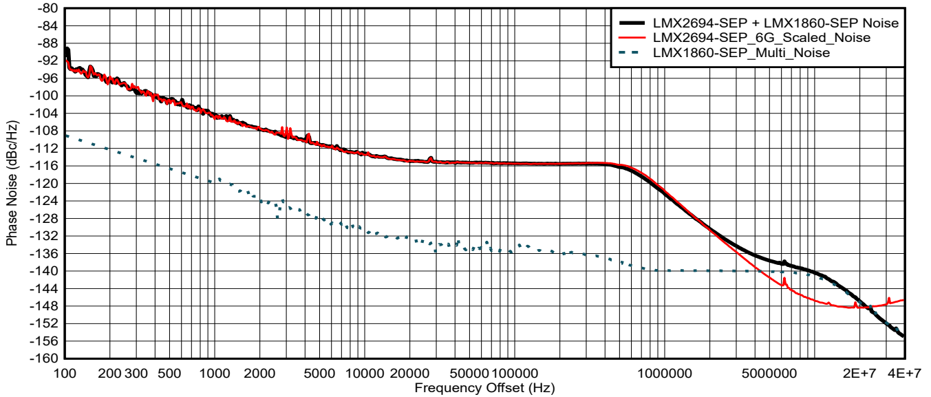
☒ 7-9. LMX1860-SEP Multiplier Output
