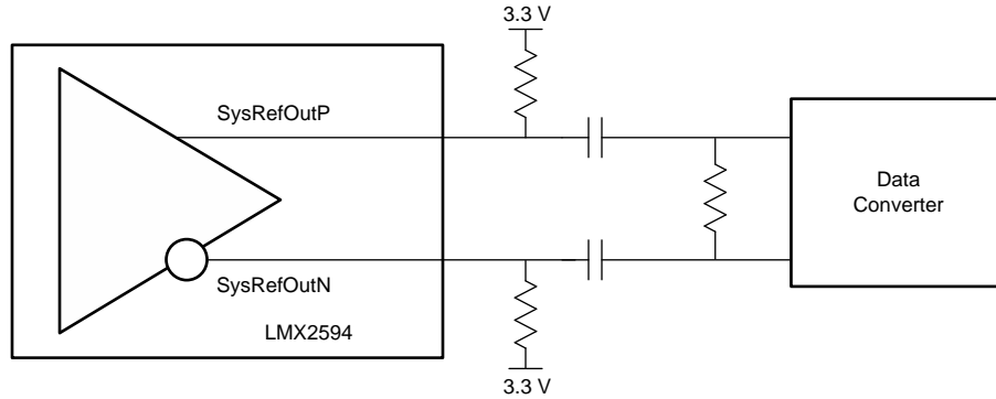
FIG 28. SYSREF Output
