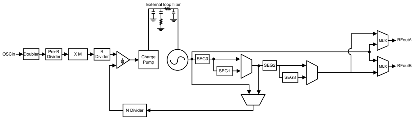
图 25. Phase SYNC Diagram
