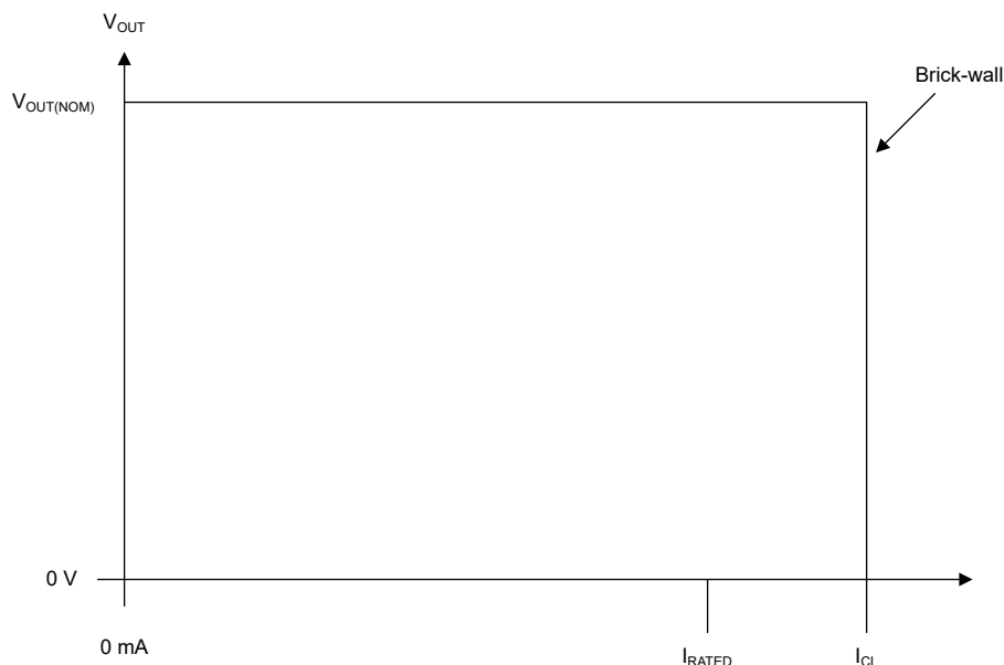
図 6-1. Current Limit
