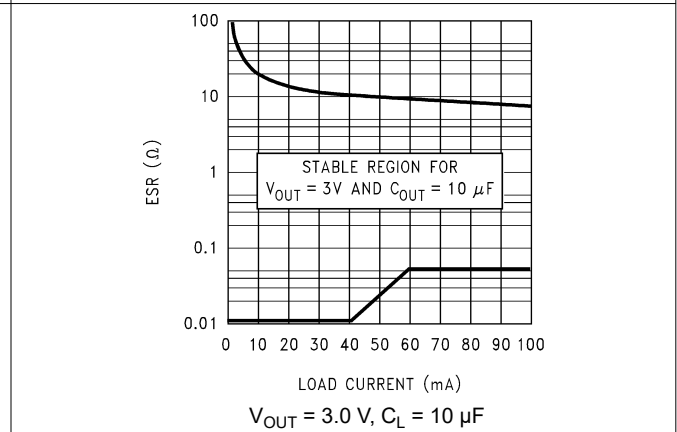
図 7-6. 3.0-V, 10- \mu F ESR Curves (Legacy Chip)
