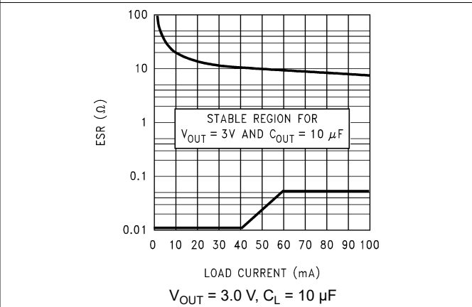
図 7-6. 3.0-V, 10- \mu\text{F} ESR Curves (Legacy Chip)
