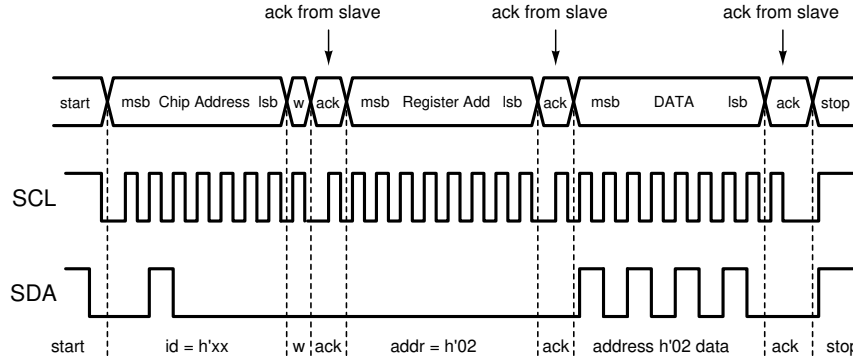
図 6-4. LP3943 Register Write
