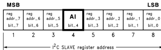
図 6-6. Register Address Byte
