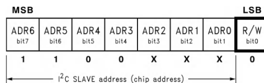
図 6-3. Chip Address Byte
