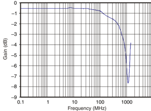
図 9-3. 3dB 帯域幅
