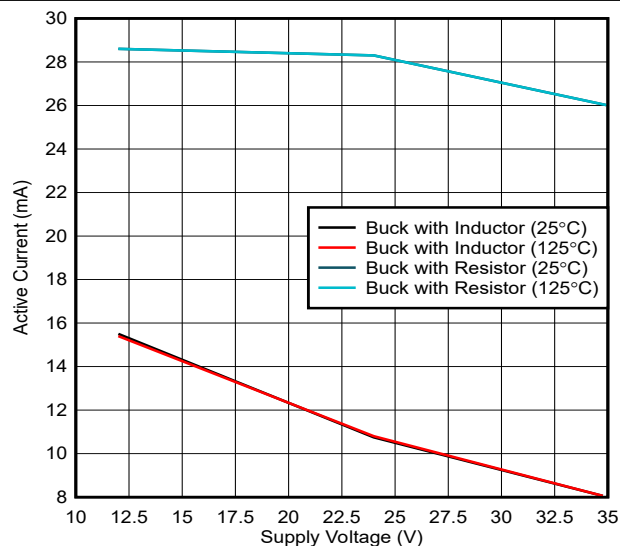
図 5-1. 電源電圧に対する電源電流
