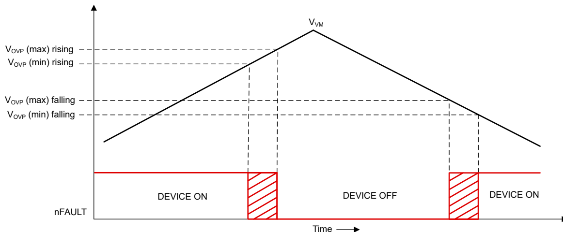
図 6-61. 過電圧保護
