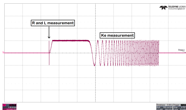
図 9-3. MPET - 相電流
