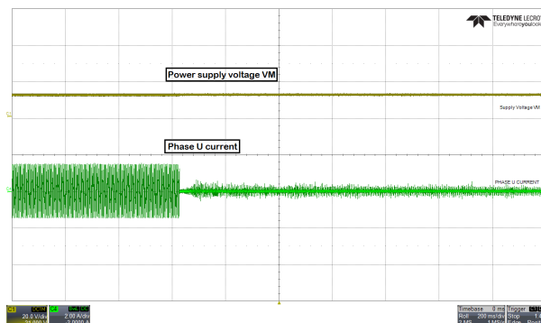
図 9-9. AVS が有効化されている場合の電源電圧と相電流の波形
