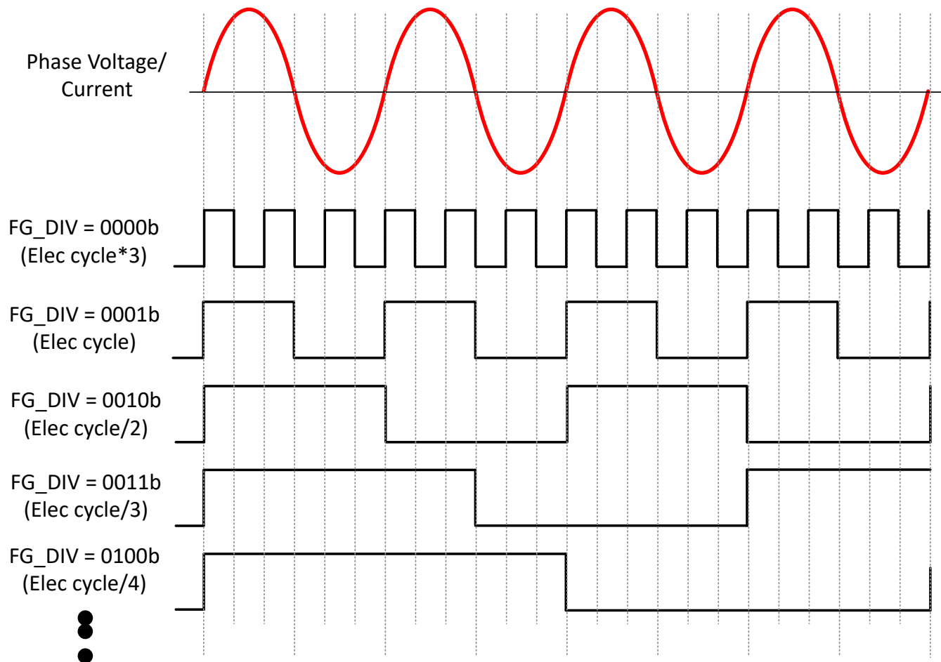
図 6-58. FG 分周器
