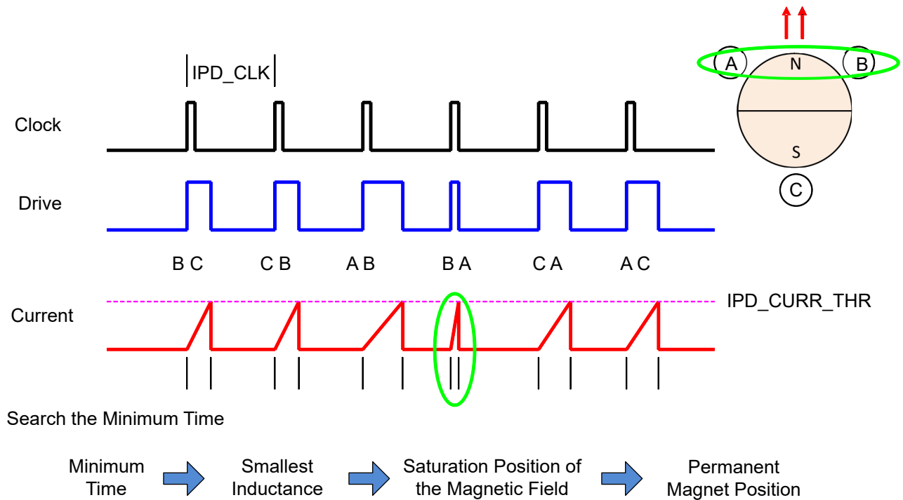
図 6-31. IPD の機能
