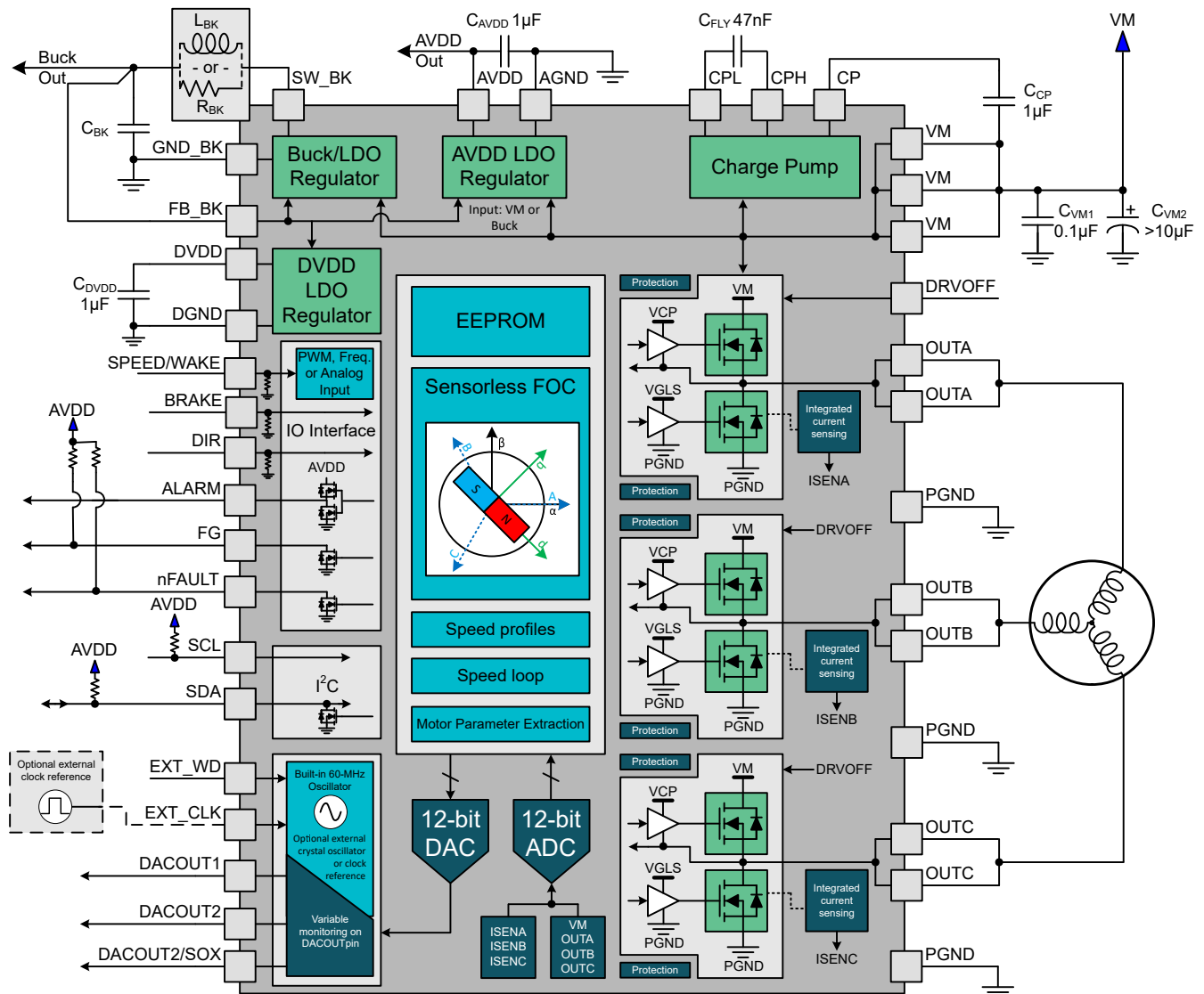
図 6-1. MCF8316D-Q1 機能ブロック図
