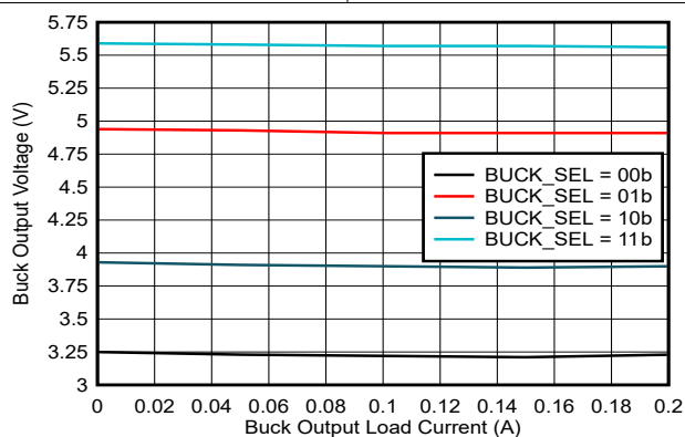
図 5-3. 負荷電流に対する降圧レギュレータの出力電圧
