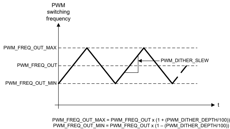
図 6-51. 三角波 PWM ディザリング
