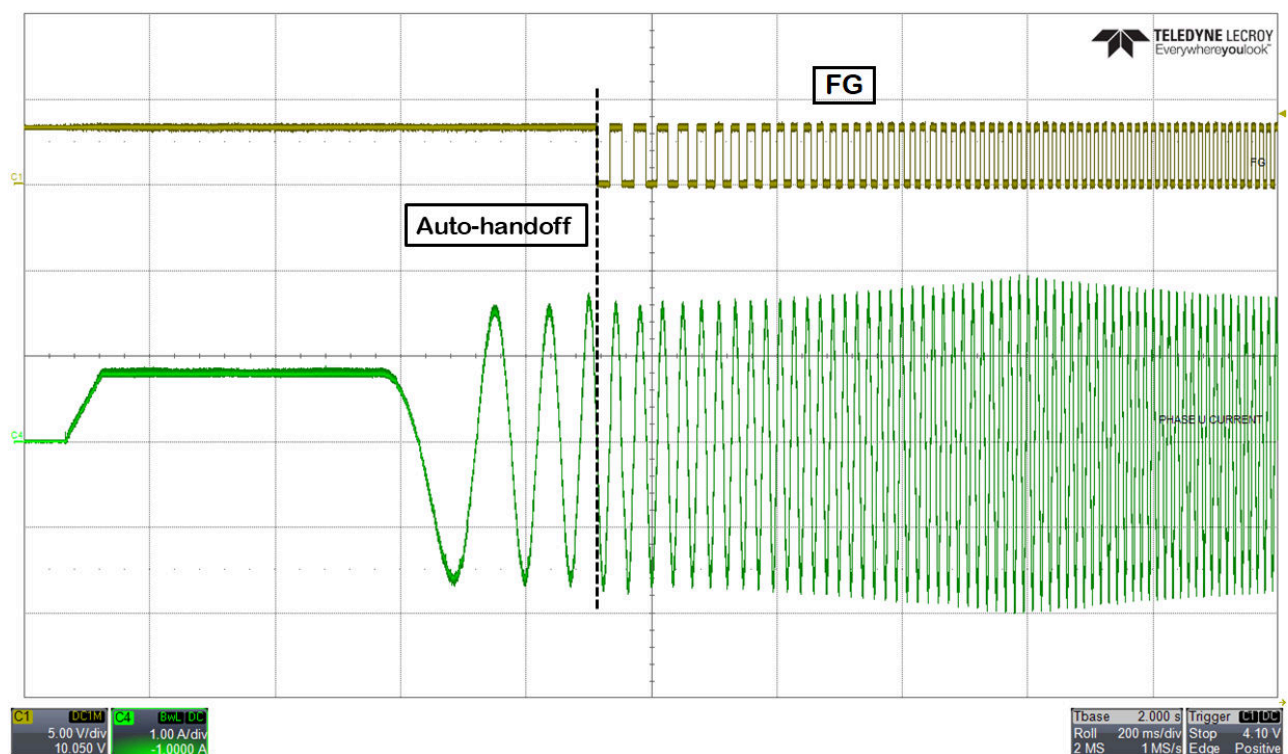
図 9-7. 自動ハンドオフ
