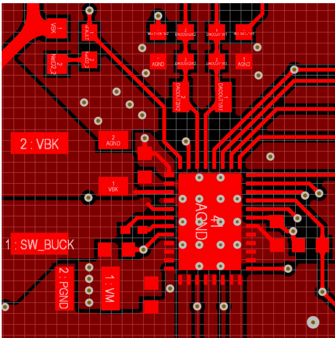
図 9-12. 推奨レイアウト例
