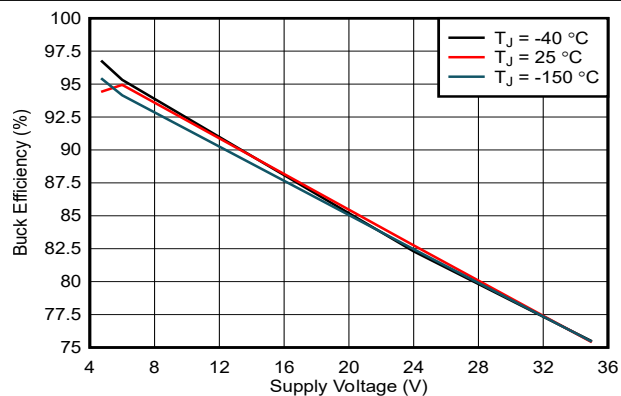
図 5-2. 電源電圧に対する降圧レギュレータの効率
