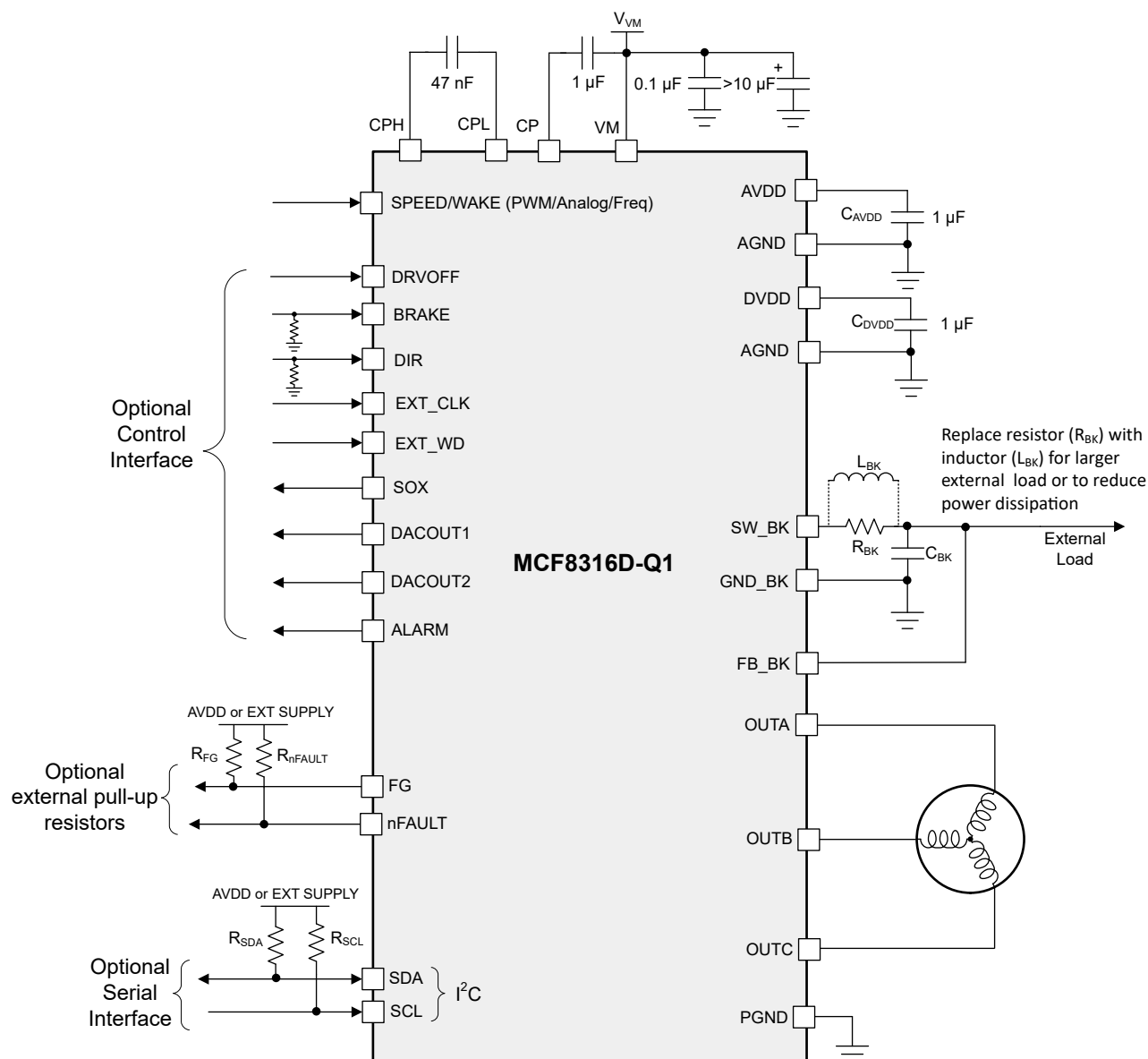
図 9-1. アプリケーションの回路図例
