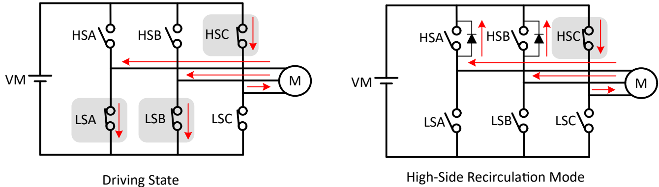
図 6-55. ハイサイド還流
