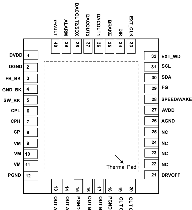
図 4-1. MCF8316D-Q1、40 ピン VQFN (露出サーマルパッド付き) 上面図
