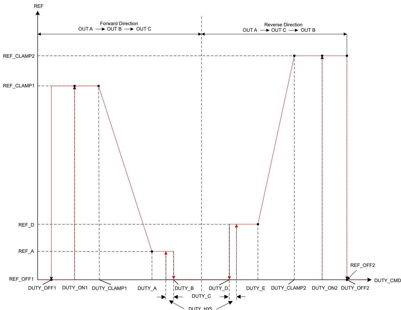
図 6-20. 双方向制御プロファイル
