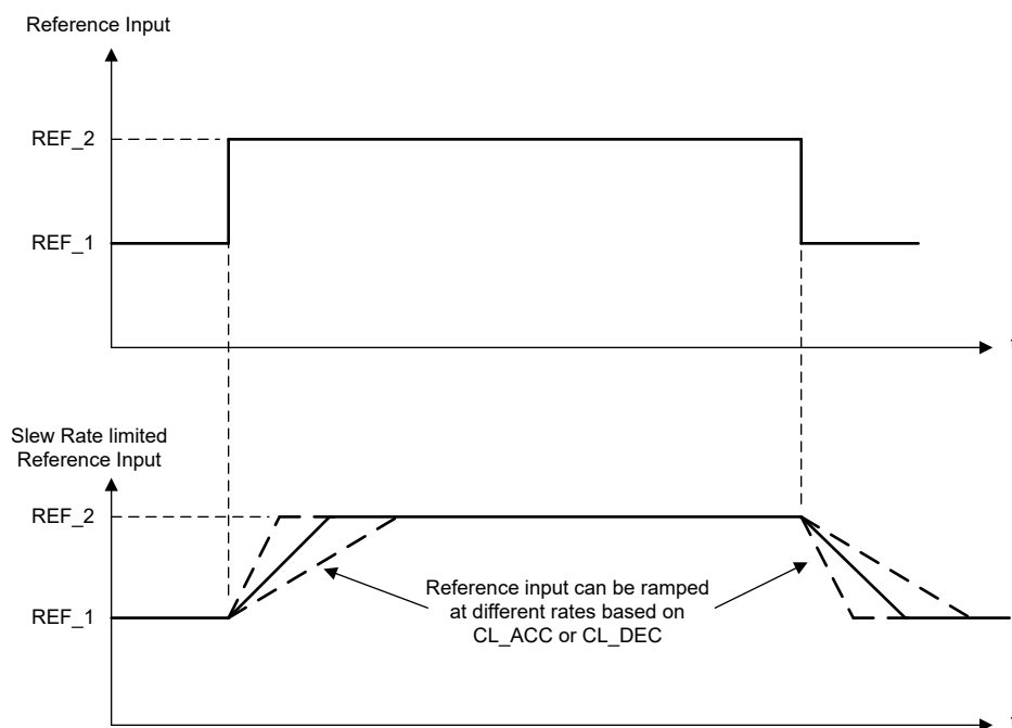
図 6-39. 閉ループ加速 / 減速スルーレート
