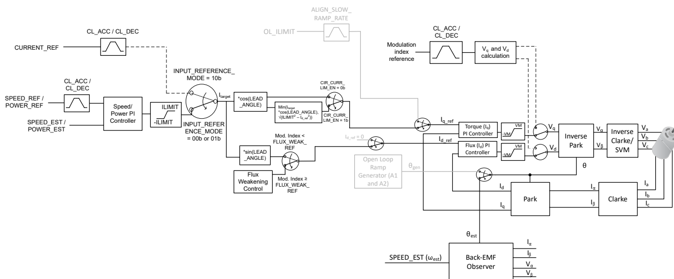
図 6-37. 開ループ - 閉ループ遷移の制御ブロック図
