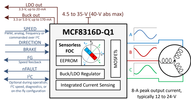
図 3-1. 概略回路図
