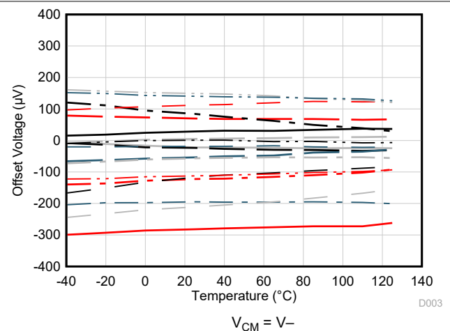
图 6-4. Offset Voltage vs Temperature
