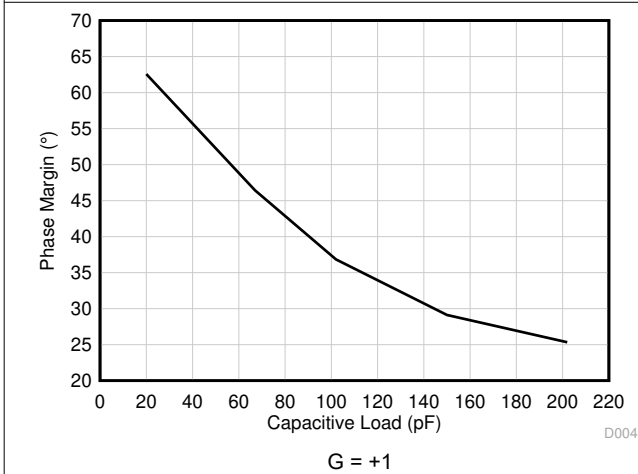
図 5-33. 位相マージンと容量性負荷との関係
