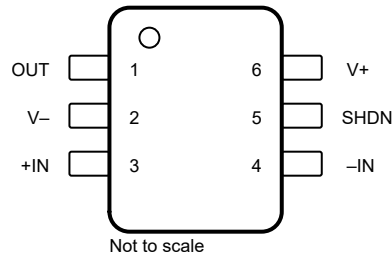
図 4-3. OPA992S DBV パッケージ 6 ピン SOT-23 (上面図)
