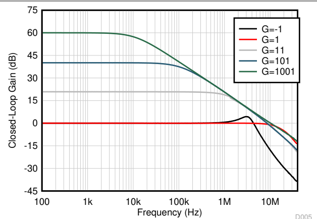
図 5-12. 閉ループゲインと周波数との関係
