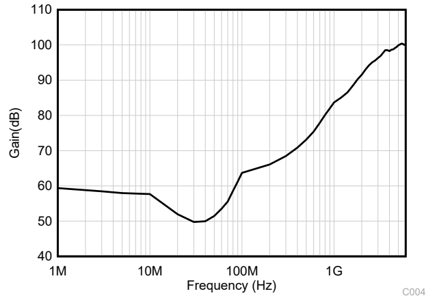
図 6-3. EMIRR Testing
