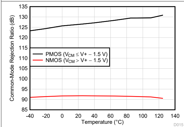
图 5-17. CMRR vs Temperature (dB)
