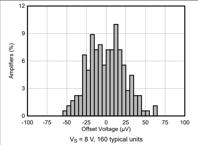
6-2. Input Offset Production Distribution
