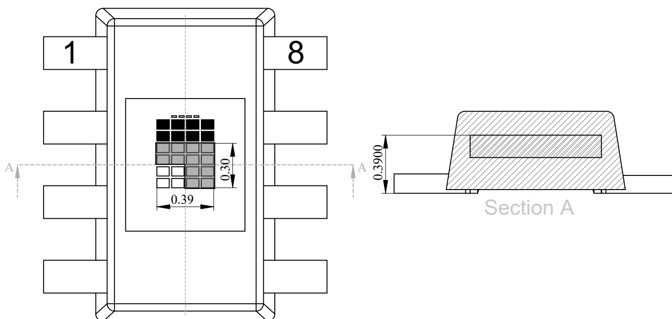
図 8-2. Sensor Position
