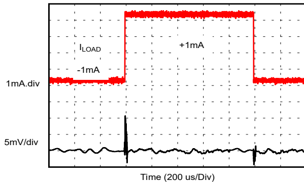
C_L = 1\mu\text{F} 、 I_{\text{OUT}} = 1\text{mA} 図 6-17. 負荷過渡
