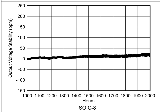
図 6-29. REF50xx の長期安定性 (2 番目の 1000 時間)
