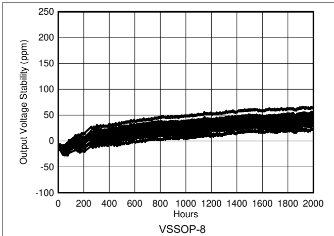
図 6-25. REF50xx の長期安定性 (最初の 2000 時間)
