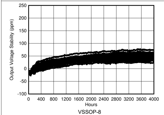
図 6-27. REF50xx の長期安定性 (4000 時間)
