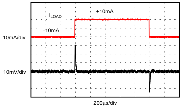
C_L = 1\mu\text{F} 、 I_{\text{OUT}} = 10\text{mA} 図 6-18. 負荷過渡
