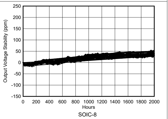
図 6-30. REF50xx の長期安定性 (2000 時間)
