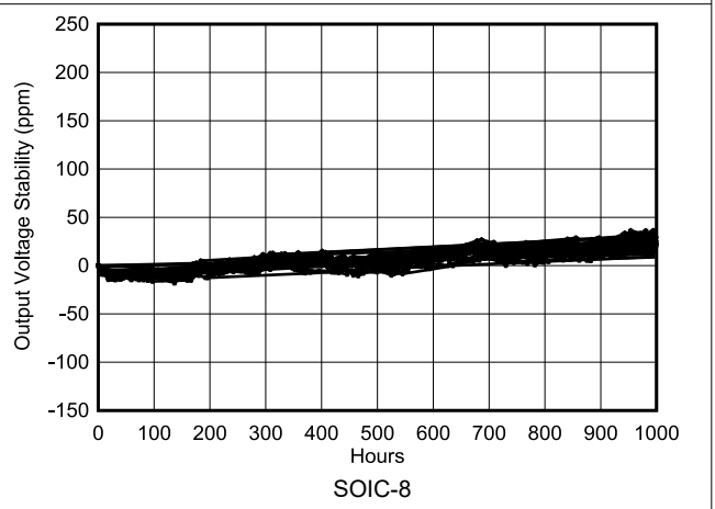
図 6-28. REF50xx の長期安定性 (最初の 1000 時間)
