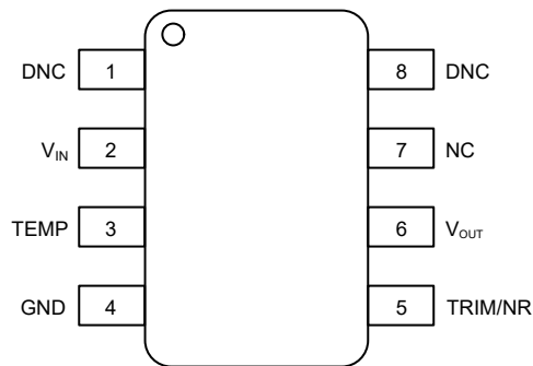
図 5-1. REF50xxAI, REF50xxID, DGK パッケージ 8 ピン SOIC、VSSOP 上面図
