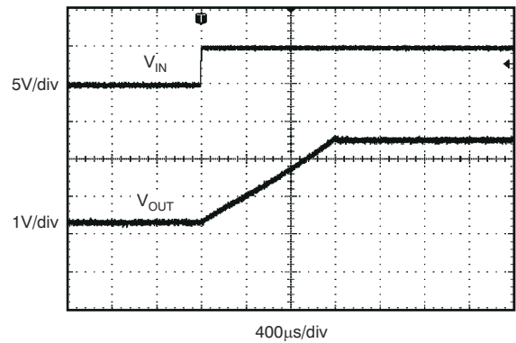
REF5025、 C_L = 10\mu\text{F} 図 6-16. スタートアップ
