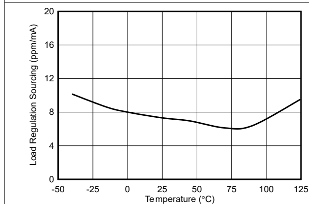
図 6-35. ロードレギュレーション (ソース) と温度との関係
