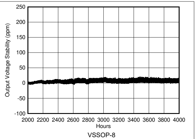
図 6-26. REF50xx の長期安定性 (2 番目の 2000 時間)
