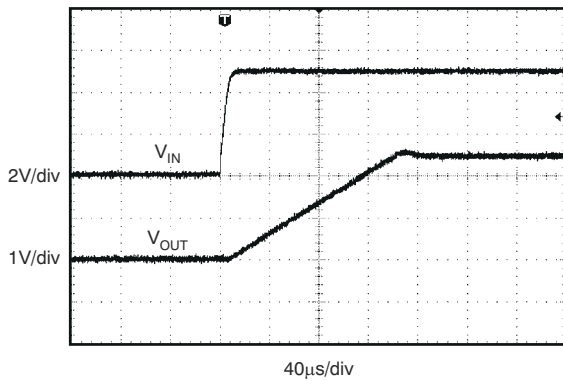
REF5025、 C_L = 1\mu\text{F} 図 6-15. スタートアップ
