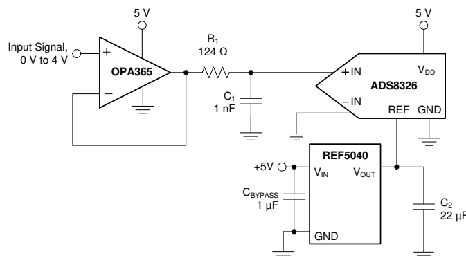
概略回路図
