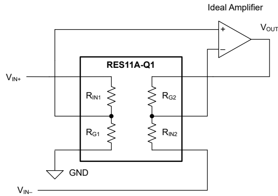
图 6-4. CMRR Calculation Reference Schematic
