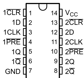
図 4-1. SN54AHC74 J または W パッケージ、14 ピン CDIP または CFP (上面図)
