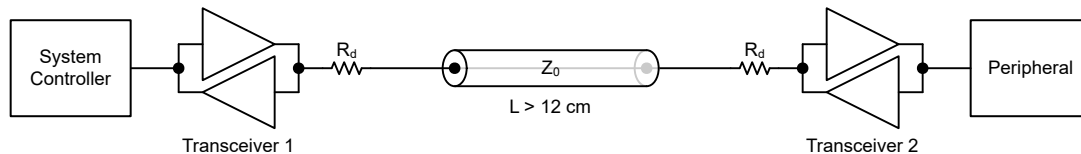
図 9-1. 代表的なアプリケーション回路図
