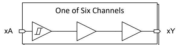
概略ロジック図
