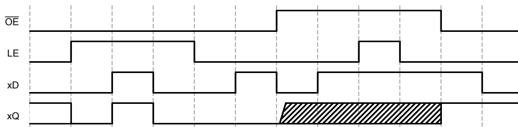
図 8-2. アプリケーション タイミング図
