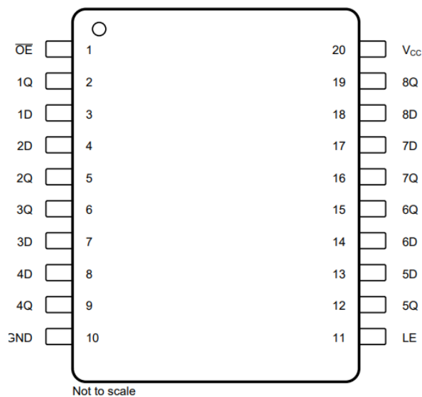
図 4-1. PW、20 ピン TSSOP (上面図)
