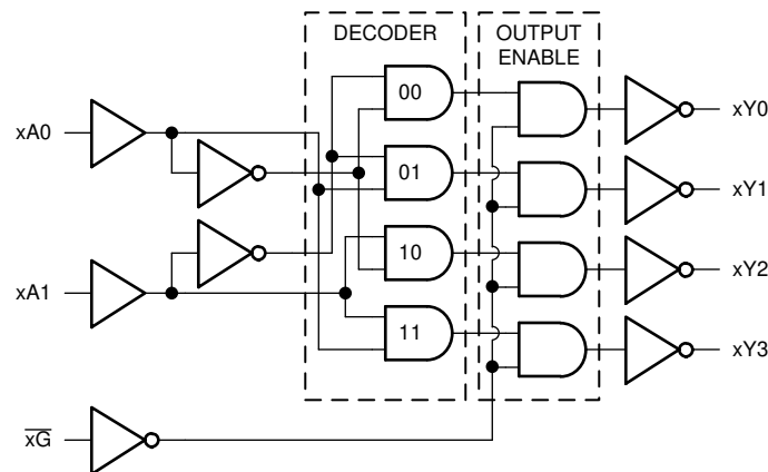
機能図
