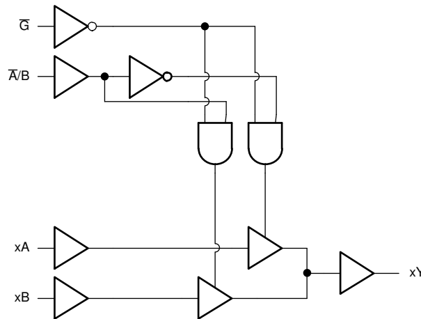
図 7-1. SN74AC157-Q1 の論理図 (正論理)
