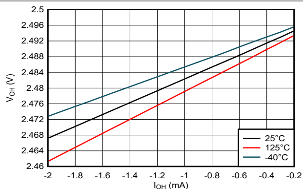
図 5-11. High 状態における出力電圧と電流との関係、2.5V 電源
