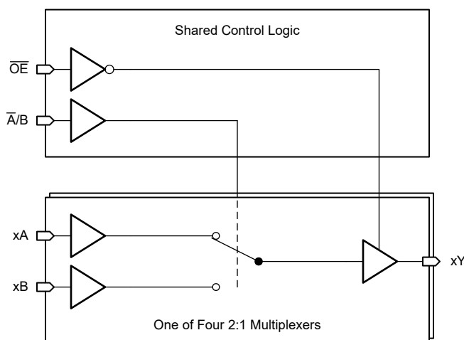
ロジック図
