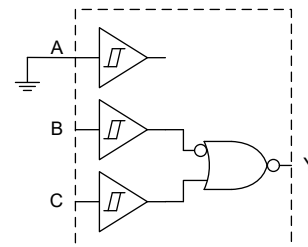
1 個の反転入力採用 2 入力 NOR
