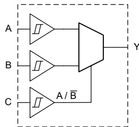
2 : 1 データ セレクタ
