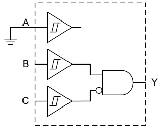
1 個の反転入力採用 2 入力 AND
