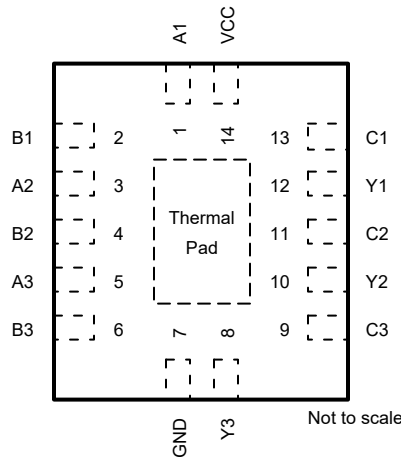
図 4-1. SN74AC3G97 BQA パッケージ、14 ピン WQFN (上面図)
