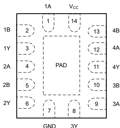
図 4-1. SN74ACT09-Q1 BQA または パッケージ (上面図)
