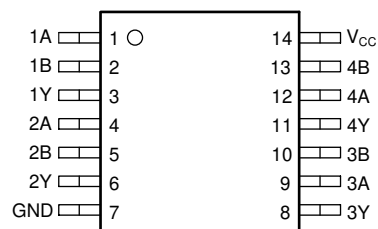
図 4-2. SN74ACT132、PW パッケージ (上面図)
