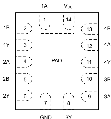
図 4-1. SN74ACT132 BQA または パッケージ (上面図)
