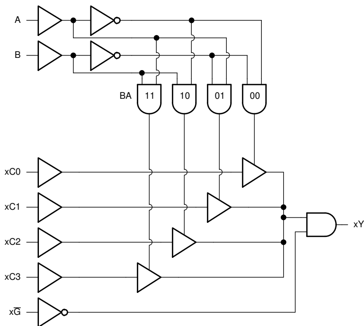
図 7-1. SN74ACT153-Q1 の論理図 (正論理)
