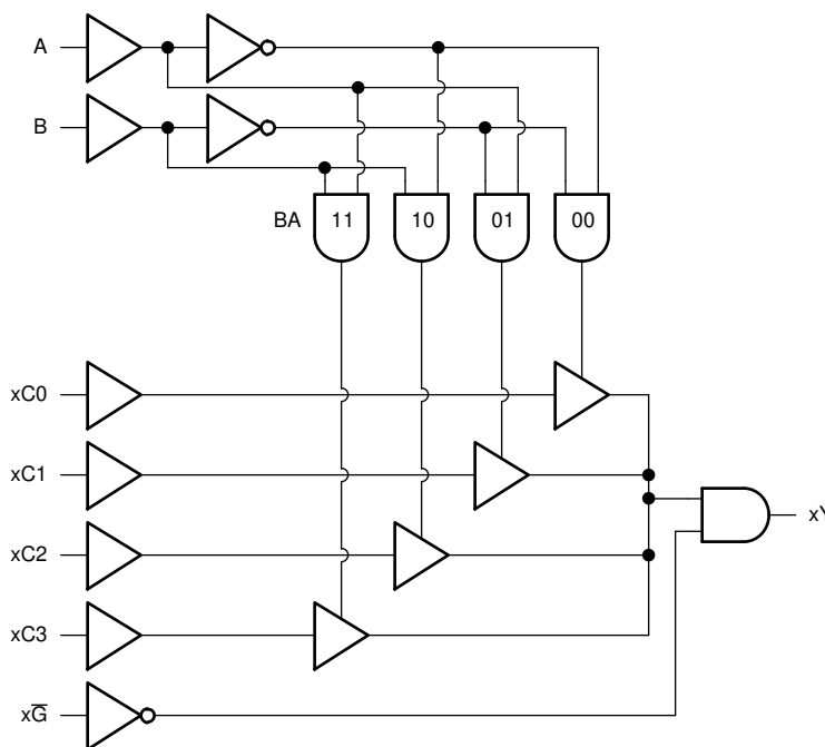
ロジック図
