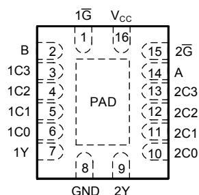
BQB パッケージ、16 ピン WQFN (上面図)
