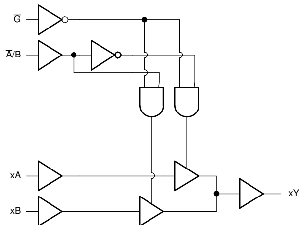
図 7-1. SN74ACT157-Q1 の論理図 (正論理)
