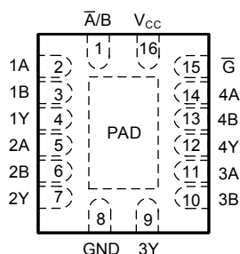
図 4-2. BQB パッケージ、16 ピン WQFN (上面図)
