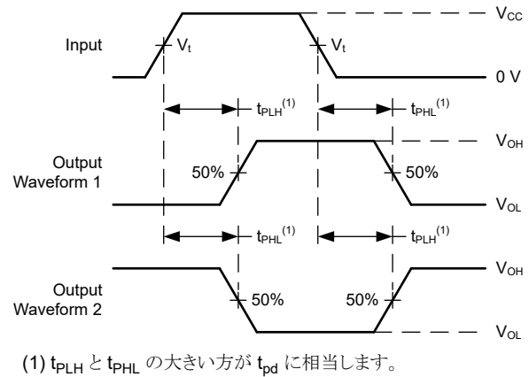
図 6-2. 電圧波形、伝搬遅延
