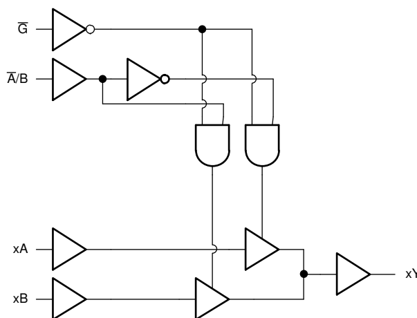
ロジック図
