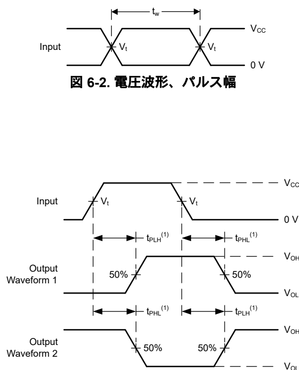
図 6-4. 電圧波形、伝搬遅延
