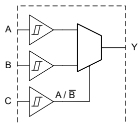
2 : 1 データ セレクタ
