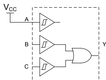
2 入力 OR ゲート
