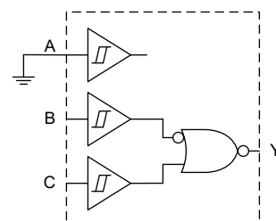
1 個の反転入力採用 2 入力 NOR
