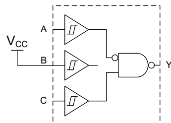
1 個の反転入力採用 2 入力 NAND
