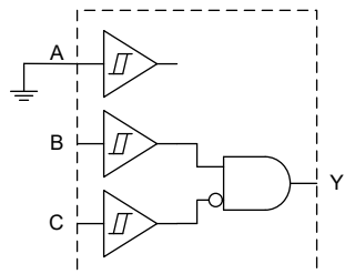
1 個の反転入力採用 2 入力 AND
