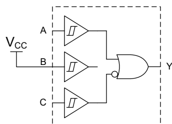
1 個の反転入力採用 2 入力 OR
