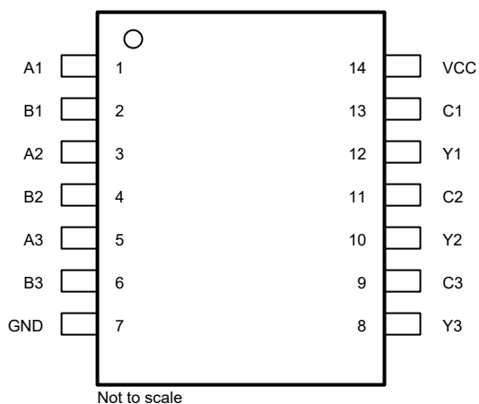
図 4-1. SN74ACT3G97 PW パッケージ、14 ピン TSSOP (上面図)
