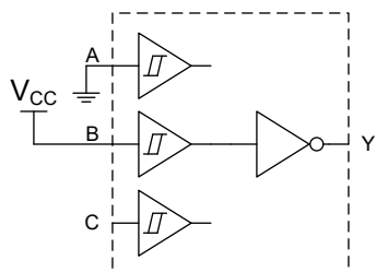
シュミットトリガインバータ
