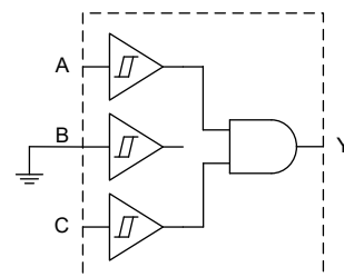
2 入力 AND ゲート
