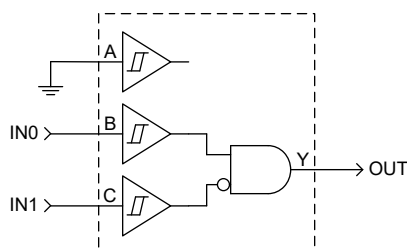
図 8-1. 代表的なアプリケーション回路図
