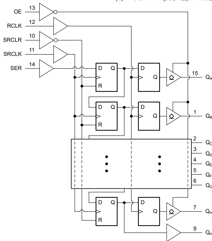
機能図
