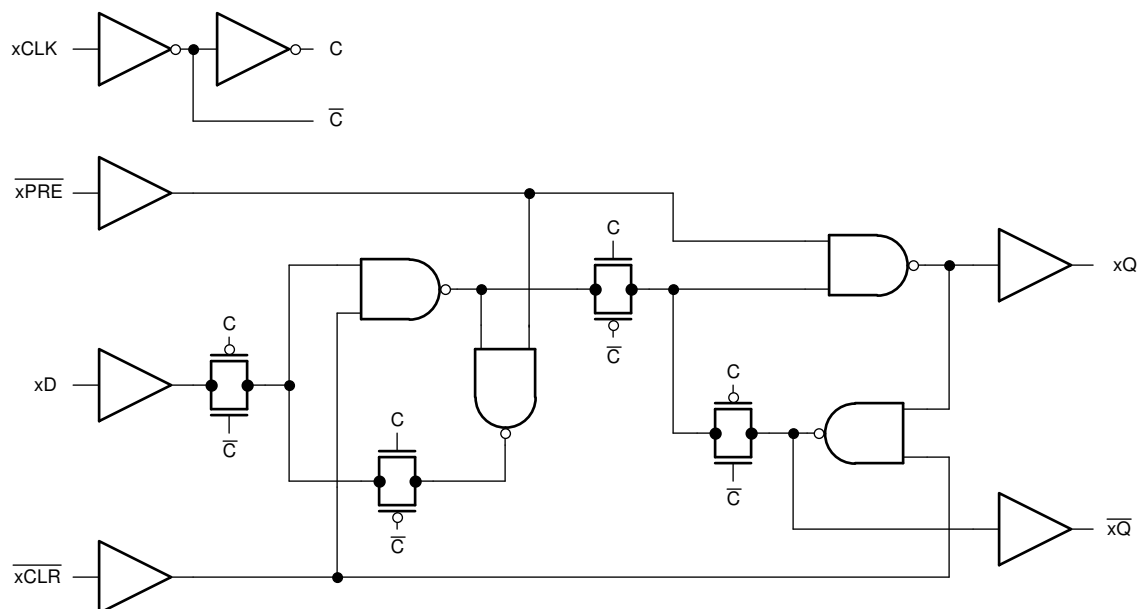
図 7-1. SN74ACT74-Q1 の 1 チャンネルの論理図 (正論理)
