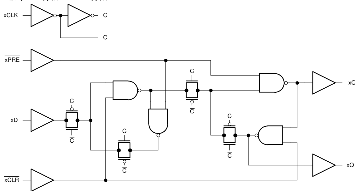
各チャネルの論理図
