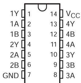
図 4-1. PW Package (Top View)
