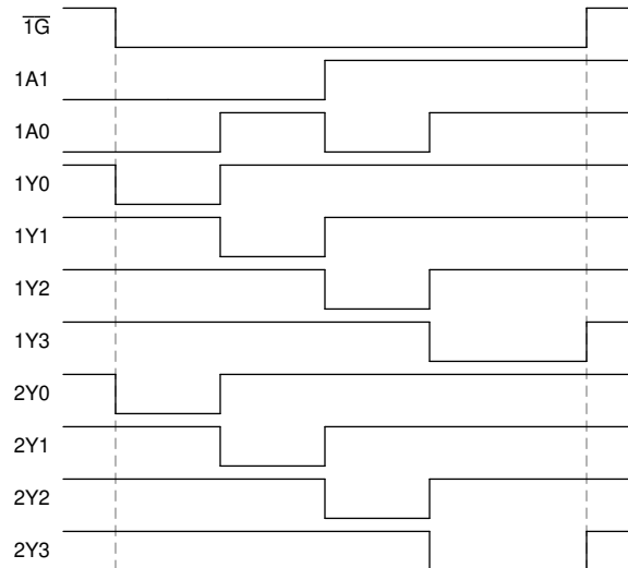
図 8-2. アプリケーション タイミング図
