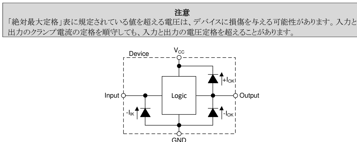
図 7-3. 各入力と出力に対するクランプ ダイオードの電気的配置
