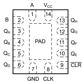
図 4-2. BQA パッケージ 16 ピン WQFN 上面図
