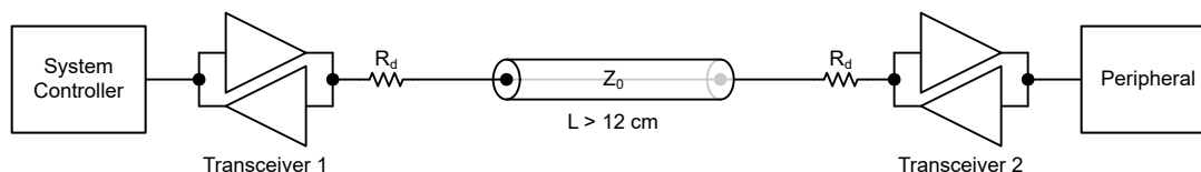
図 8-1. アプリケーション ブロック図
