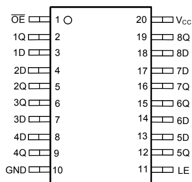
図 4-2. SN74AHC373-Q1 PW、DGS パッケージ (上面図)
