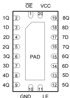
図 4-1. SN74AHC373-Q1 RKS パッケージ (上面図)
