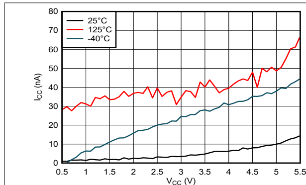
図 5-1. 電源電流と電源電圧との関係
