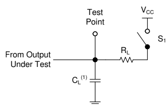
図 6-1. オープン ドレイン出力の負荷回路
