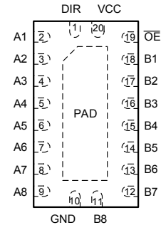
図 5-2. SN74AHCT245: RGY or RKS Package, 20-Pin VQFN (Top View)
