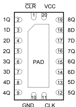
図 4-1. SN74AHCT273-Q1 RKS または RGY パッケージ (上面図)
