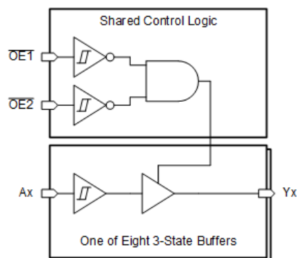
図 7-1. シュミット トリガ入力図
