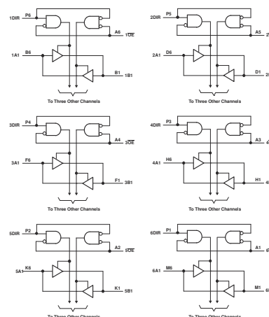
図 3-1. ロジック図
