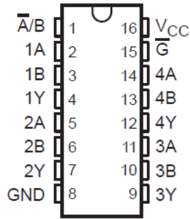
J、D、DB、N、NS、PW パッケージ 16 ピン CDIP、SOIC、SSOP、PDIP、SO、TSSOP 上面図
