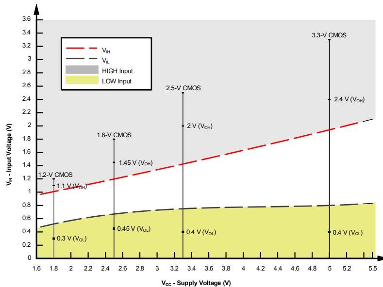
図 7-2. SCxT の 電圧レベル
