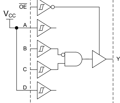
1 個の反転入力採用 2 入力 AND
