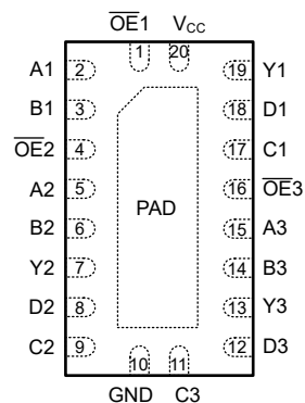
図 4-1. PW または DGS パッケージ、20 ピン TSSOP 図 4-2. RKS パッケージ、20 ピン VQFN (透過上面図) または VSSOP (上面図)
