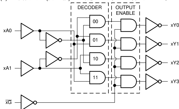
論理図 (正論理)
